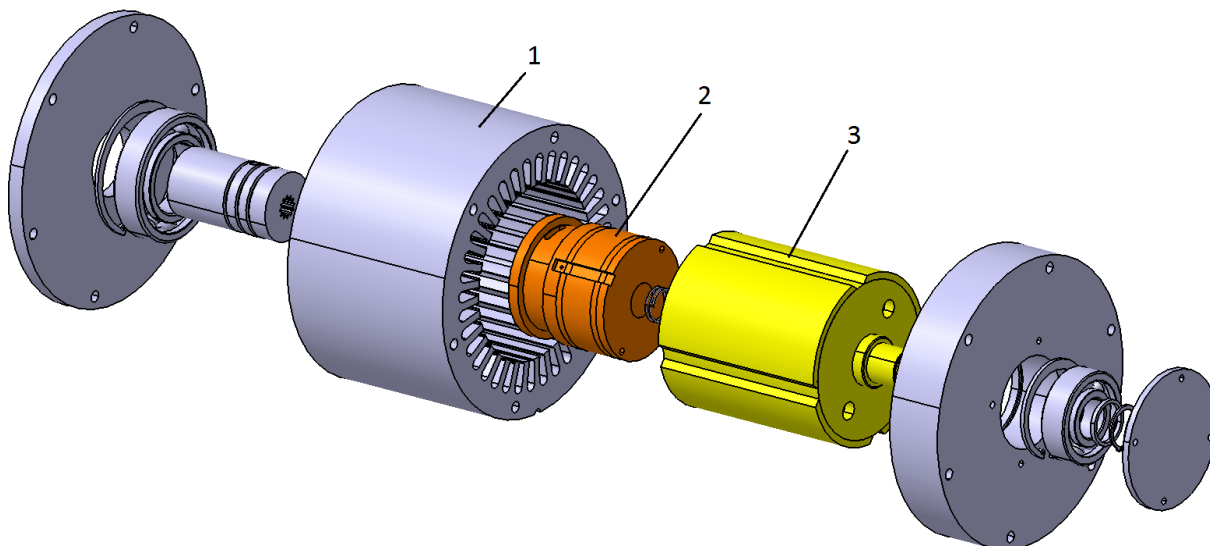
Rys. 3. Zespół silnik-pompa
