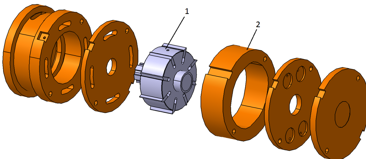
Rys. 4. Zespół pompy łopatkowej
