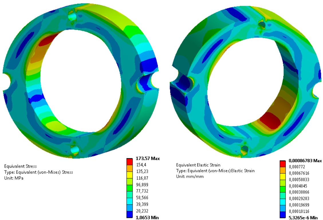
Rys. 9. Naprężenia [MPa] i odkształcenia [mm] zredukowane wg hipotezy Hubera-Misesa bieźni pompy łopatkowej.
