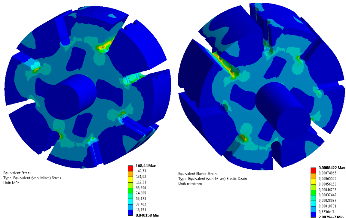
Rys. 8. Naprężenia [MPa] i odkształcenia [mm] zredukowane wg hipotezy Hubera-Misesa wirnika pompy łopatkowej.
