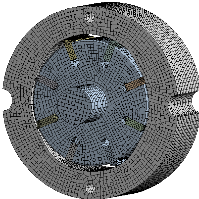
Rys. 5. Model MES pompy łopatkowej
