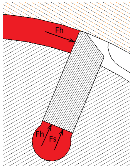
Rys. 6. Obciążenia od ciśnienia działające na łopatkę oraz siła pochodząca od sprężyn.
