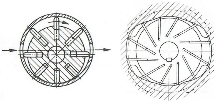
Rys. 1. Schematy pomp pojedynczego i podwójnego działania.
