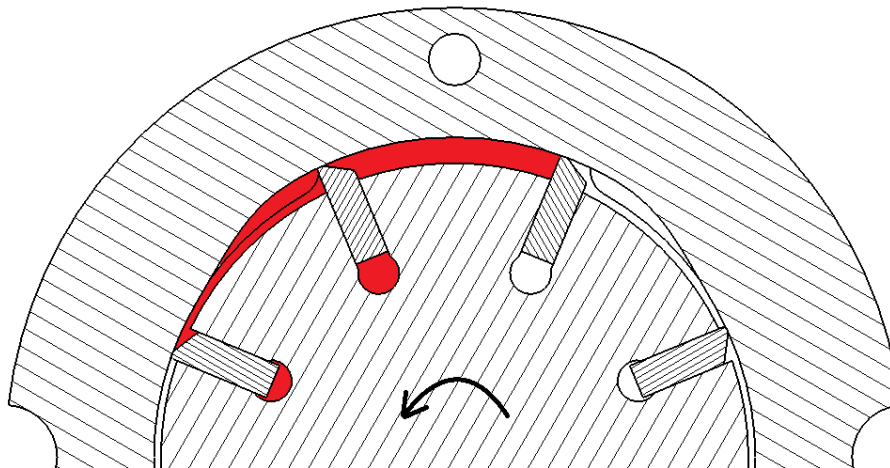
Rys. 7. Rozkład ciśnienia w pompie
