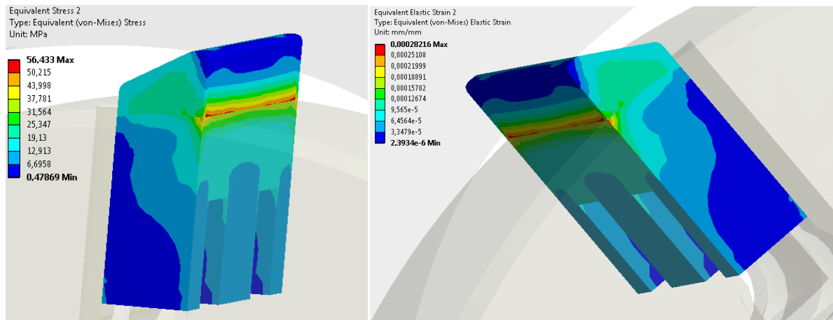
Rys. 10. Naprężenia [MPa] i odkształcenia [mm] zredukowane wg hipotezy Hubera-Misesa łopatki pompy łopatkowej.
